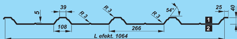
PROFIL DACHOWY
