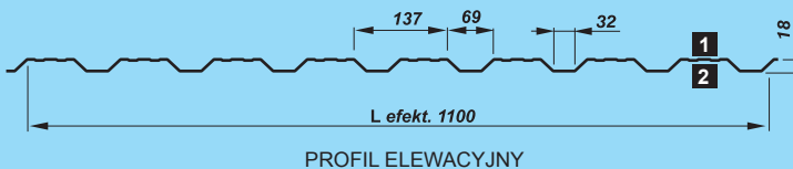
PROFIL ELEWACYJNY
