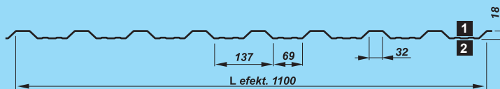
PROFIL DACHOWY
